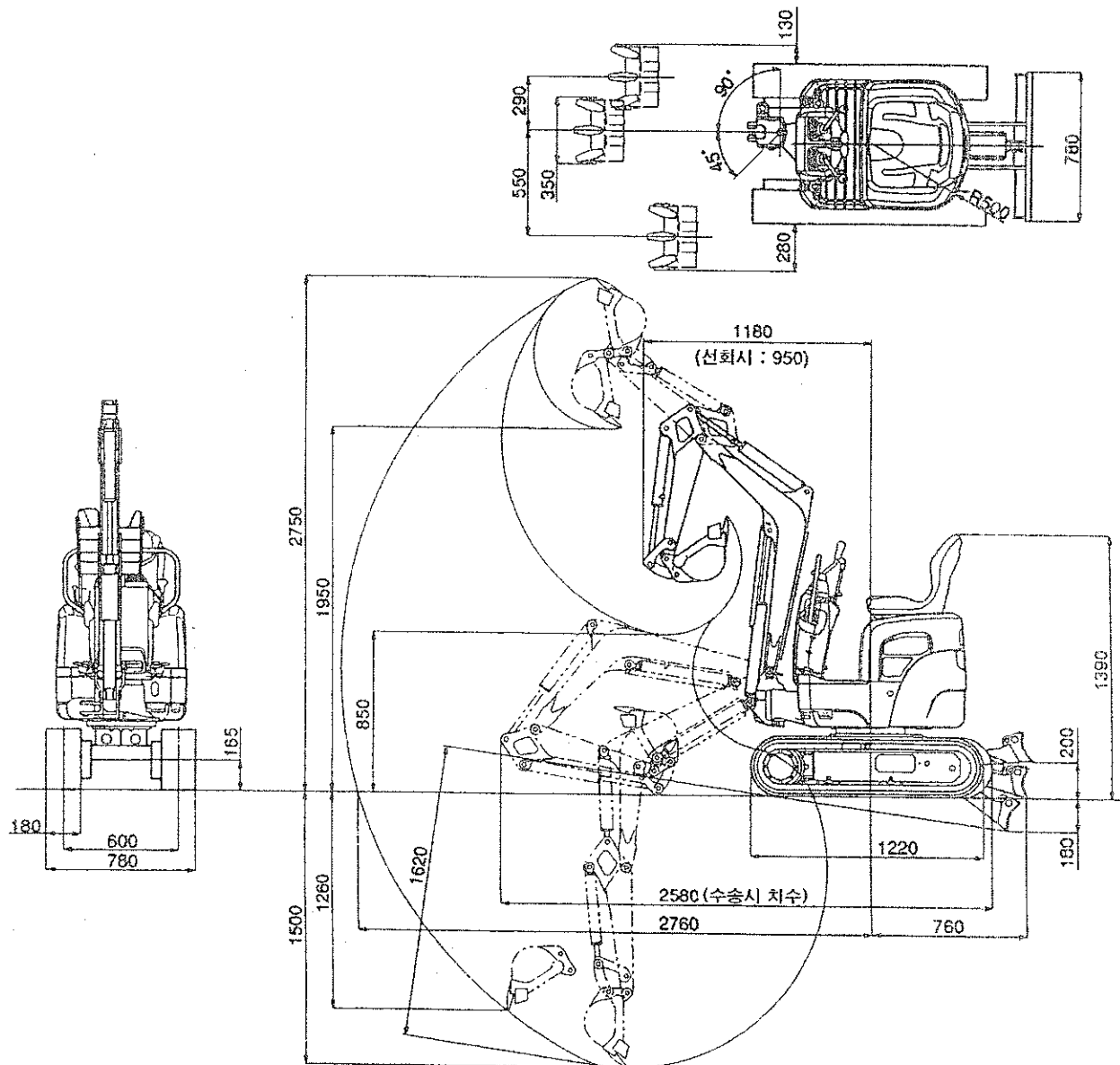
트랙폭 고정식 장비의 외형도
