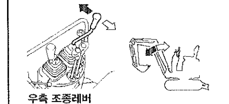
■ 버킷 조작
